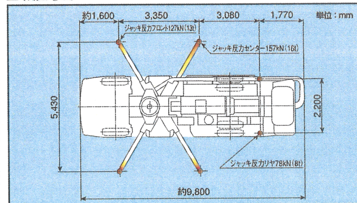
■ 設置寸法
